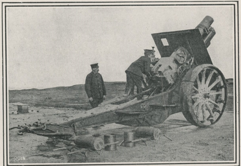
OBUSIER DE 8' T. R. SCHNEIDER
